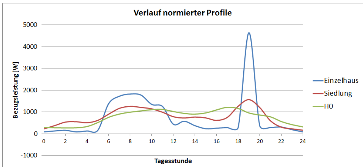
Abbildung 1: Zeitlicher Verlauf der Bedarfsprofile exemplarisch für Einzelhaustyp A, Siedlung und übergeordnetes Netz (H0) an einen typischen Wochentag.
